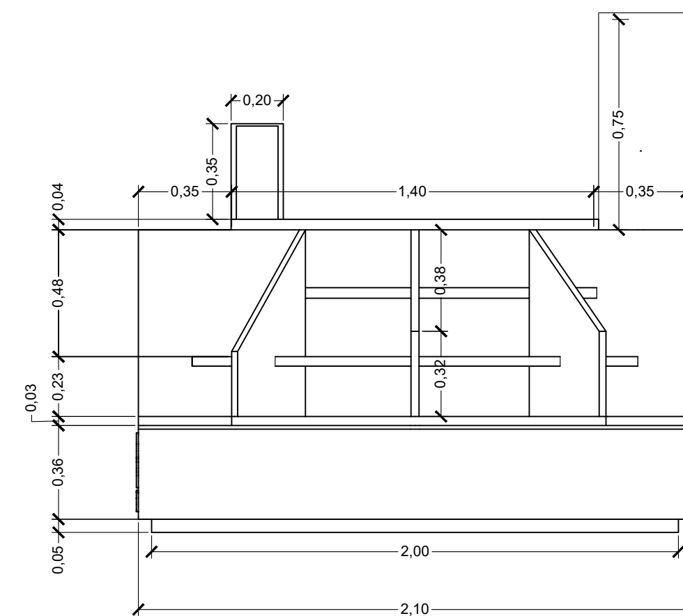
VISTA LATERAL DERECHA - ISLA PETITE AFFAIRE ESC. 1.20
