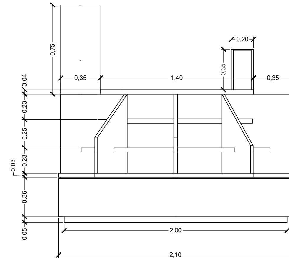
VISTA LATERAL IZQ - ISLA PETITE AFFAIRE ESC. 1.20
